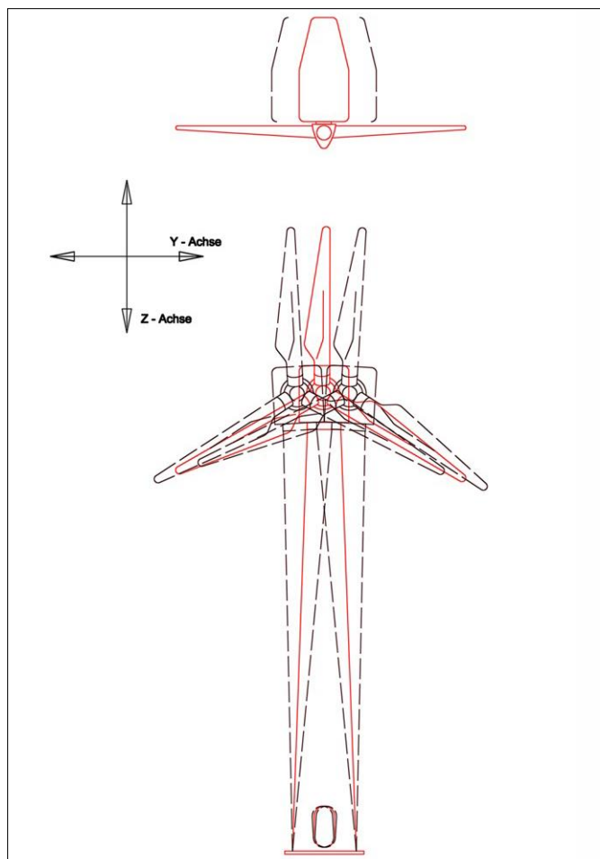
Schwingungen einer Windenergieanlage
